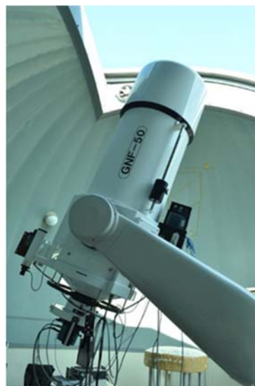
図 2：大阪教育大学天文台の口径 51cm 反射式望遠鏡
