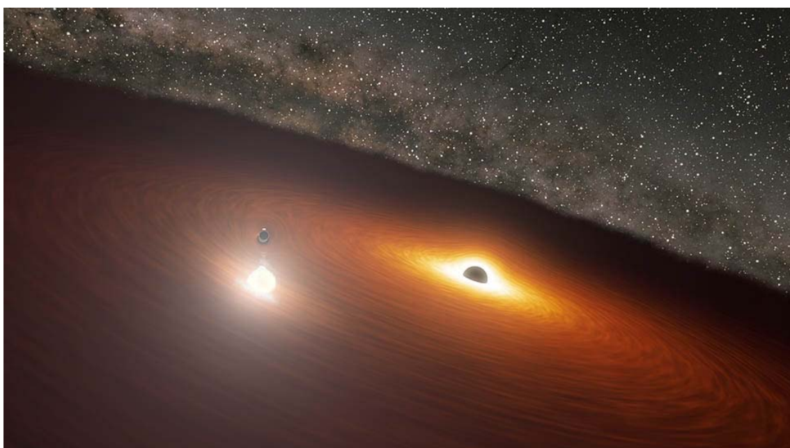
図 3 : OJ 287 の連星ブラックホールの想像図。右の中心のブラックホールを、左の衛星ブラックホールが約 12 年周期で公転運動しています。中心のブラックホールの周囲には降着円盤と呼ばれるガス円盤構造が存在し、衛星ブラックホールは 1 公転につき 2 回それに衝突し突き抜けることとなりますが、その際に膨大な光が発せられます。2019 年 7 月の増光は、衛星ブラックホールが地球から見て降着円盤の反対側から手前側へ突き抜けることで生じました (地球は図の上方に位置するとした構図)。(クレジット : NASA/JPL-Caltech/R. Hurt (IPAC))
