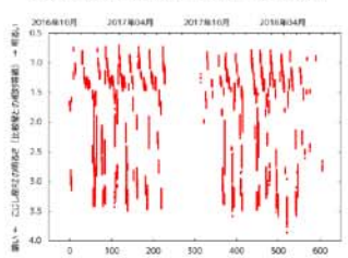
おおぐま座ER型矮新星「こじし座RZ」の光度曲線
