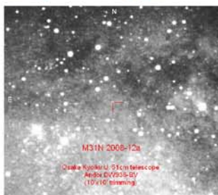
2016年に観測されたアンドロメダ銀河で爆発した新星(2本の赤い線で示した点光源)。アンドロメダ銀河の距離は約250万光年なので、この新星が実際に爆発したのは250万年前です。(51cm望遠鏡によるRCVバンド画像)
