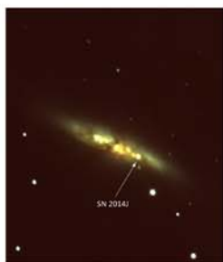
スターバースト銀河である葉巻銀河M82で発生したIa型のSN 2014J(矢印)(51cm望遠鏡による3色合成画像)
