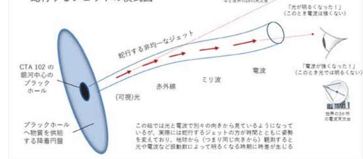
CTA 102 のブラックホールと蛇行するジェットの模式図
